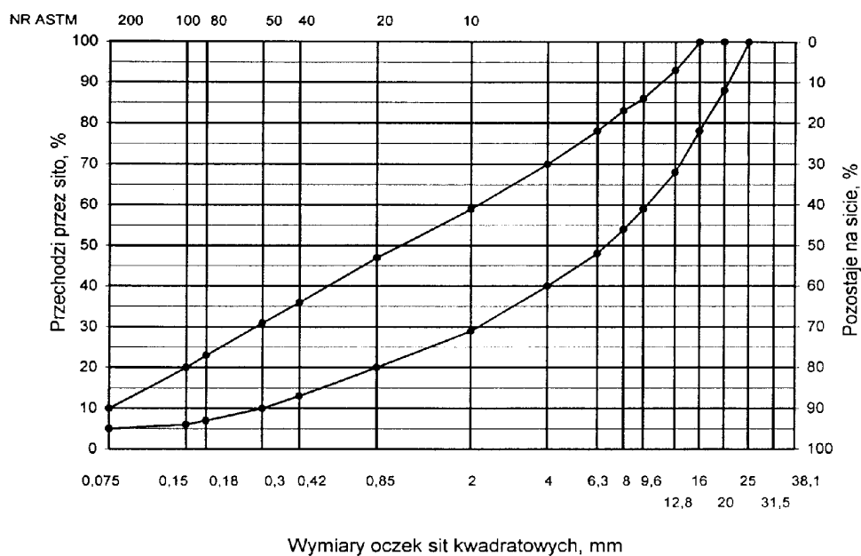
Rys. 1. Krzywe graniczne uziarnienia mieszanki mineralnej BA od 0 do 20 mm do warstwy ścieralnej nawierzchni drogi o obciążeniu ruchem dla KR2
